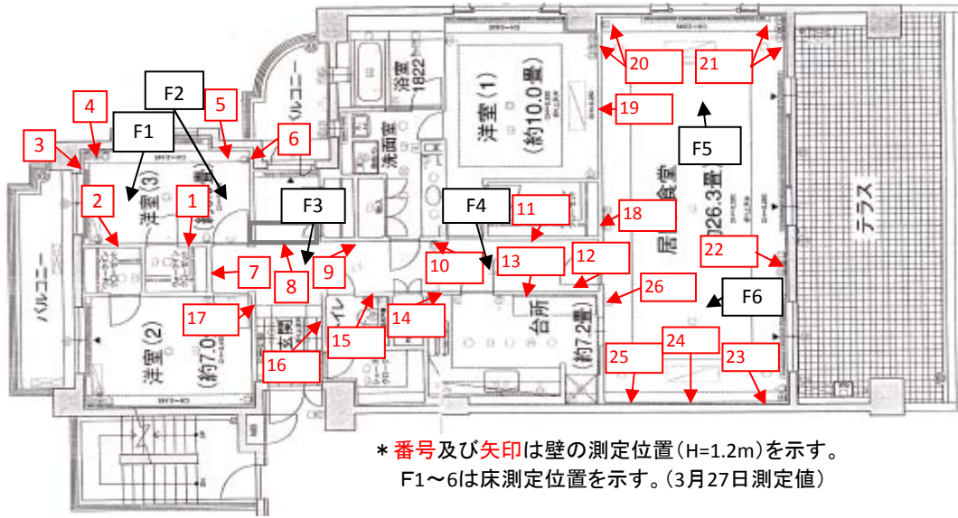
号室 平面図
